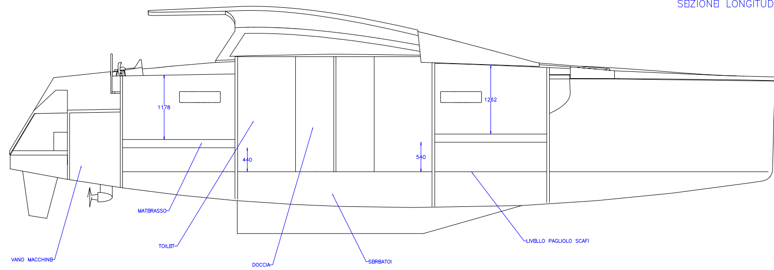
SEZIONE LONGITUDINALE @ HULL CL
